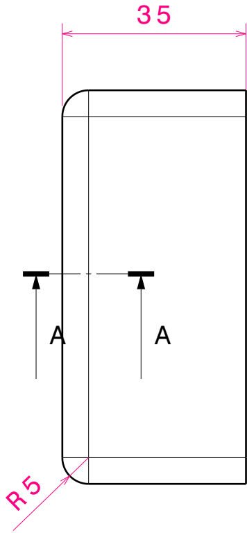
Seitenansicht rechts Maßstab: 1:1
